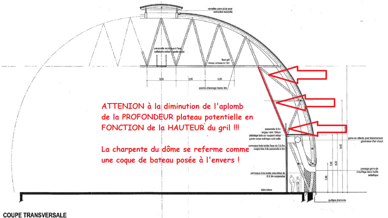
COUPE TRANSVERSALE
